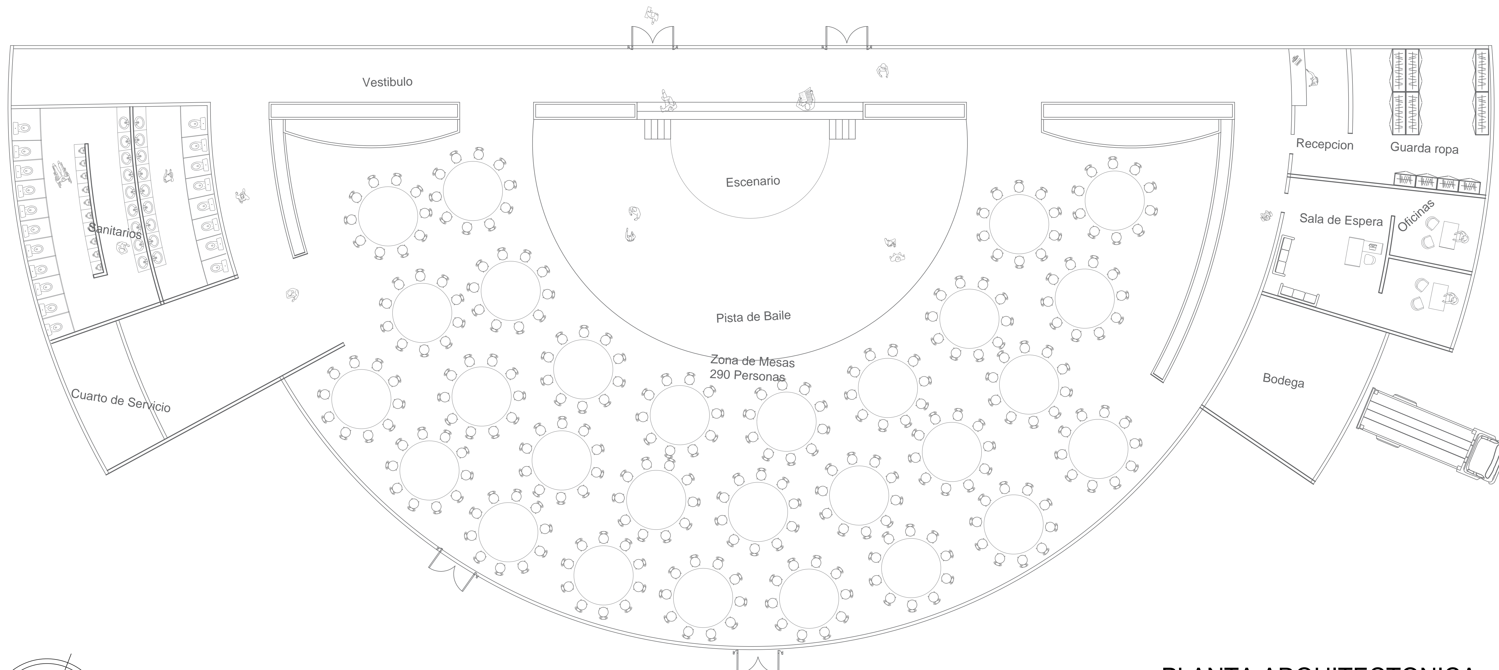
PLANTA ARQUITECTONICA SALÓN DE EVENTOS
